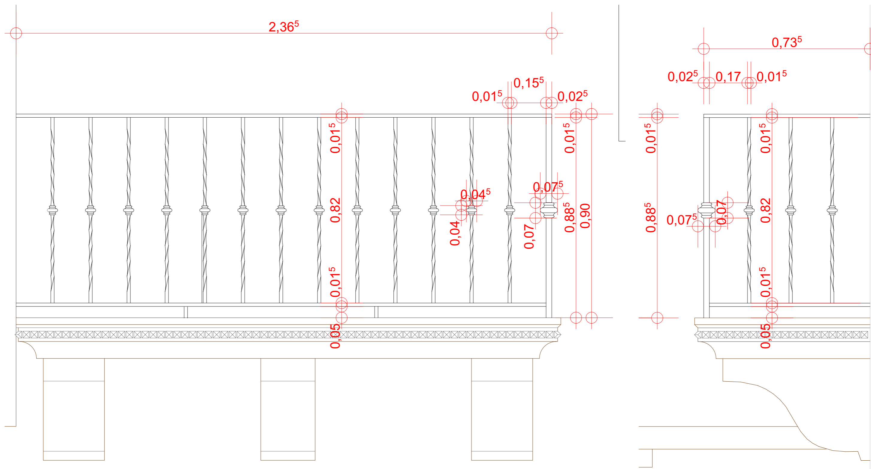
DETAJL OGRAJE NA BALKONU - PREDNJI POGLED 1:10
